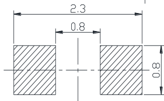
推荐焊盘尺寸
