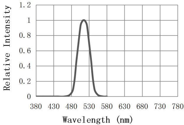
光谱分布特性曲线
