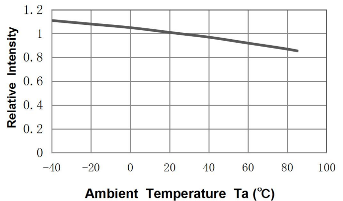
相对光强与环境温度特性曲线
