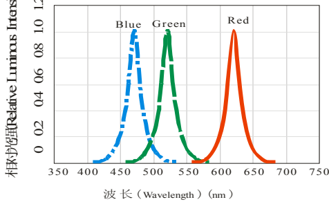
光谱分布特性曲线 Relative Spectral Distribution
