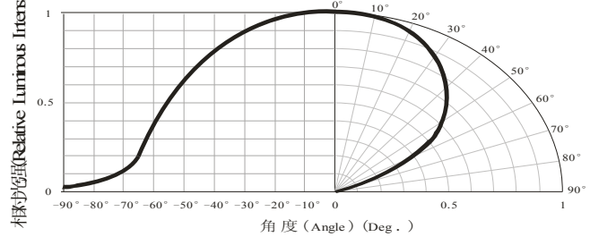
光强分布特性曲线 Typical Spatial Distribution
