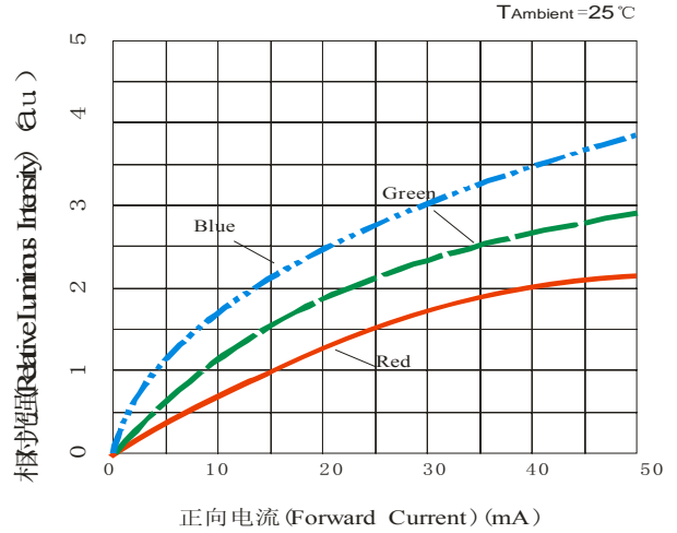
相对光强与正向电流特性 Relative Luminous Intensity VS Forward Current
